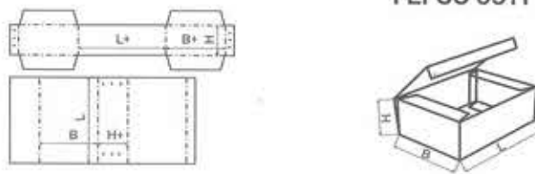
FEFCO 0511
