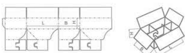
FEFCO 0718
