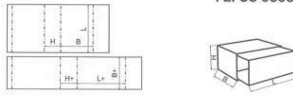
FEFCO 0507
