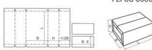
FEFCO 0607
