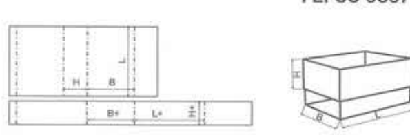
FEFCO 0508
