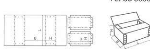
FEFCO 0606
